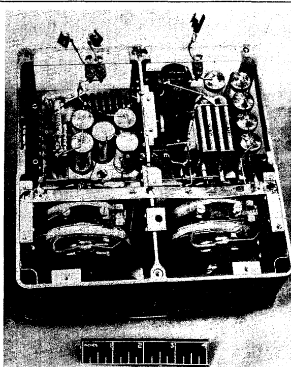
FuG 17 - FuG 17E & Z (AIRBORNE TRANS.-RECVR)
